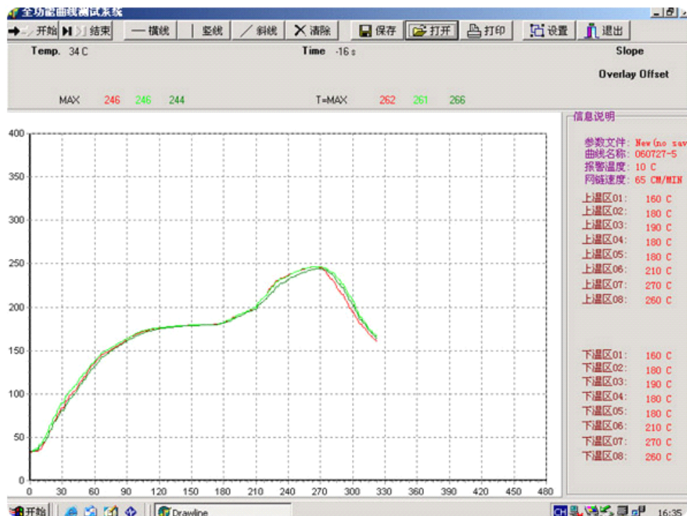
精确温度曲线测试系统（使用本公司测试 PCB 测试）
