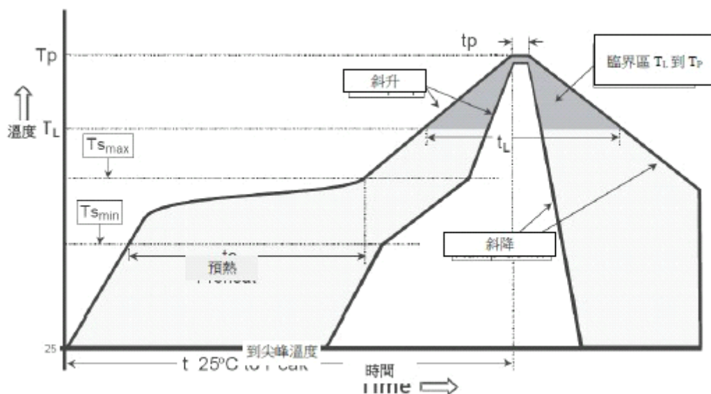
精确温度曲线测试系统（使用本公司测试 PCB 测试）
