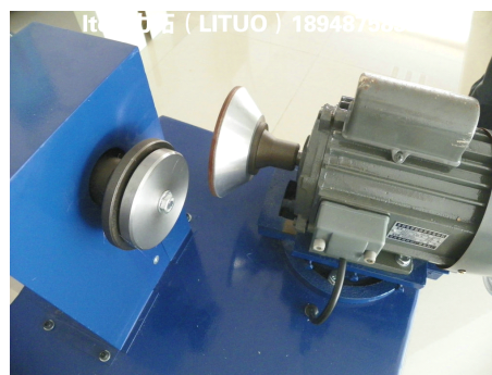
LT-250A 钨钢刀研磨装置
